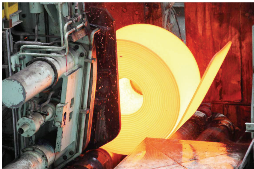
2019 年,北部湾新材料公司压延车间热轧生产线使用热卷箱将粗轧中间坯头尾对调作业现场 北部湾新材料公司 供
