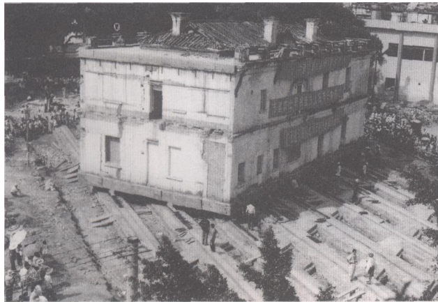
1999年10月初，原英领馆往东北方向平移55.8米。图为平移中的原英领馆
